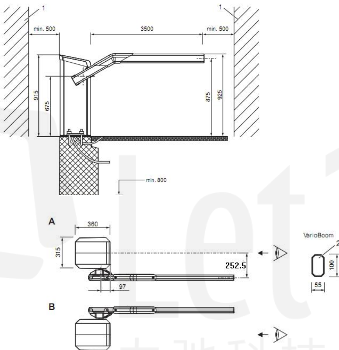
图 5：栏杆机系统尺寸和栏杆臂简介——“Parking”系列
