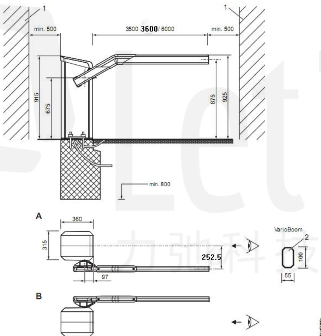
图 3: 栏杆机系统的尺寸和栏杆臂简介——“Access”系列
