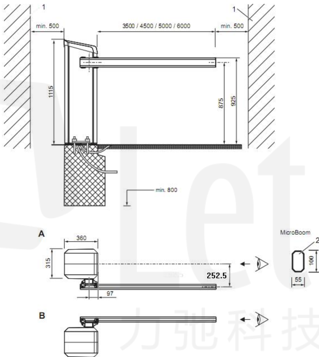
图 4：栏杆机系统和栏杆臂的尺寸简介——“Access Pro H”系列
