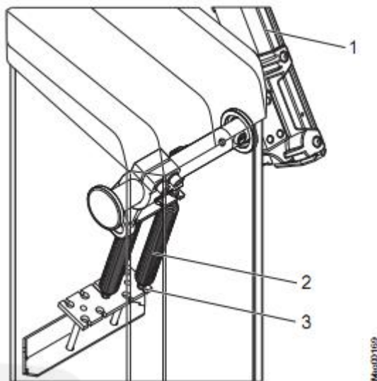
图 35: 杠杆系统的平衡弹簧
