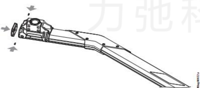
图 58: 安装端盖
