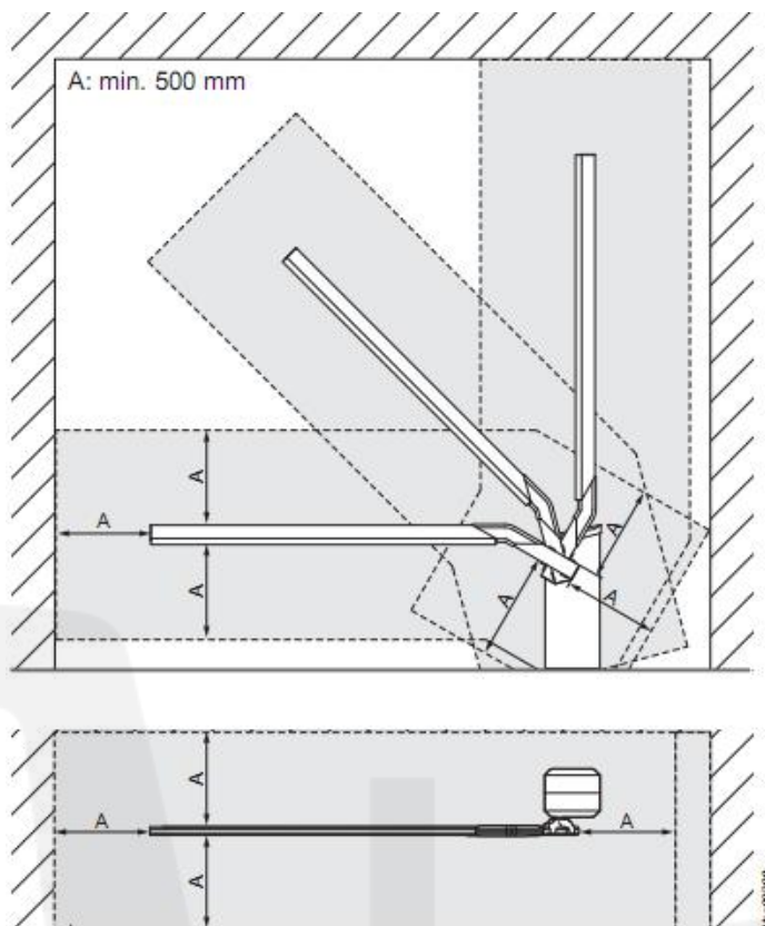
图 1：危险区域 A 500mm 的危险区
