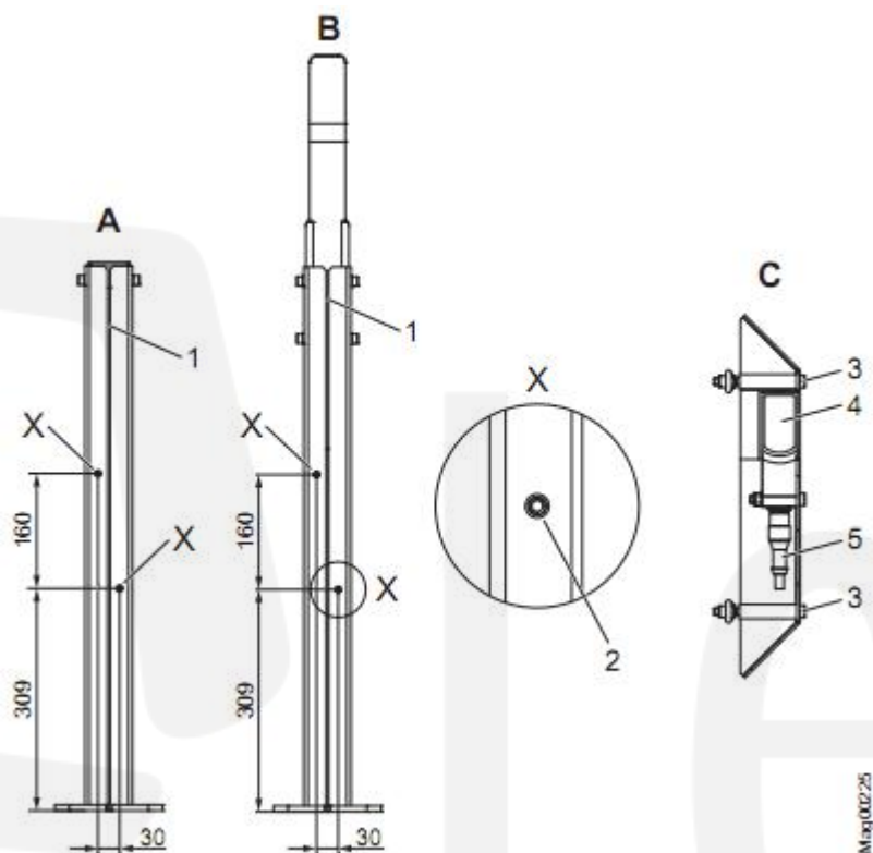
图 26：在支柱架上安装接收器的光栅机
