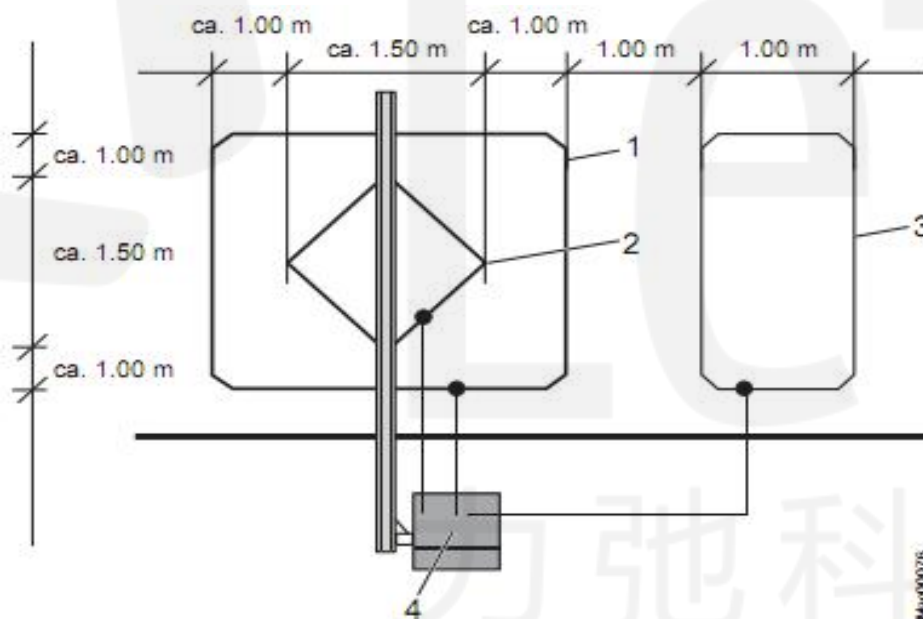
图 13: 客车/卡车感应线圈
