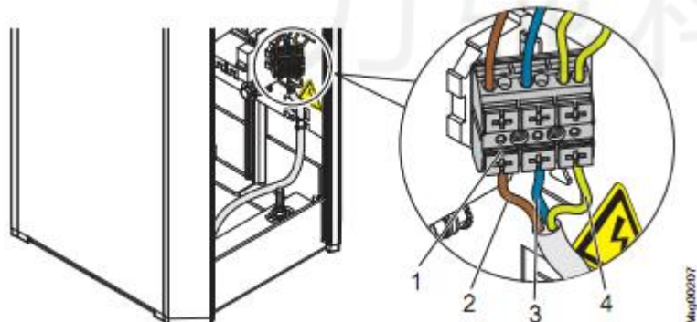
图 39: 连接电源线
