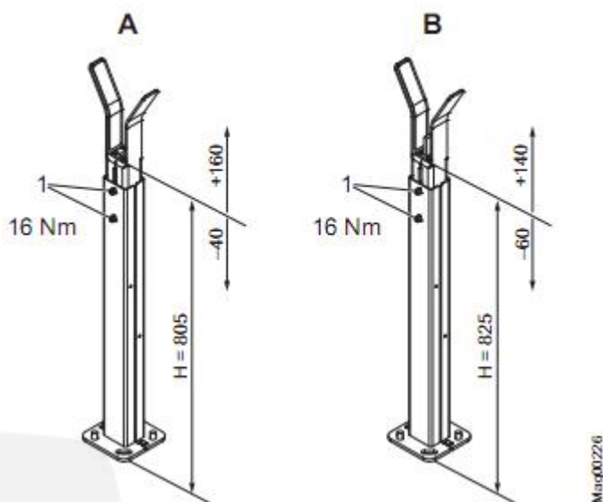
图 36: 设置嵌套支架高度
