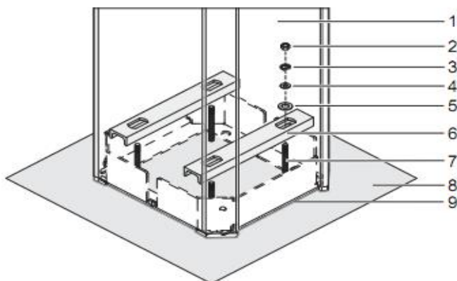
图 24: 安装栏杆机箱
