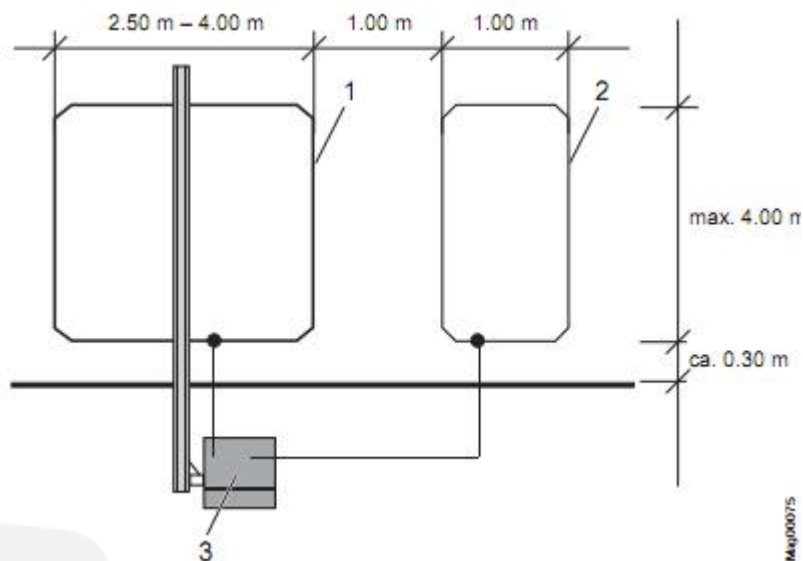
图 12 卡车感应线圈
