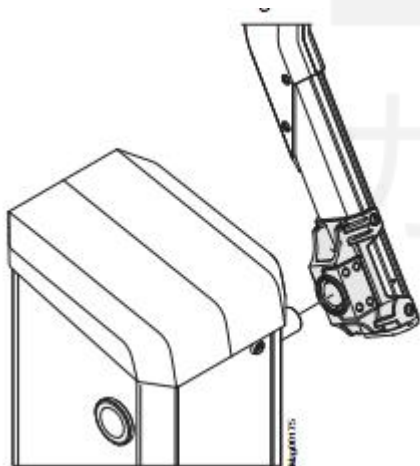
图 32：卸下回转和栏杆臂
