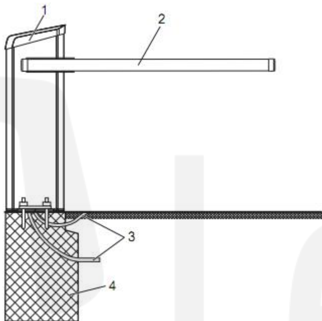
图 9: “Toll” 系列的栏杆机系统构造
