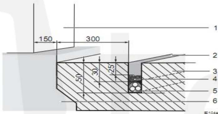
图 22: 在沥青，柏油，混凝土路面安装感应线圈
