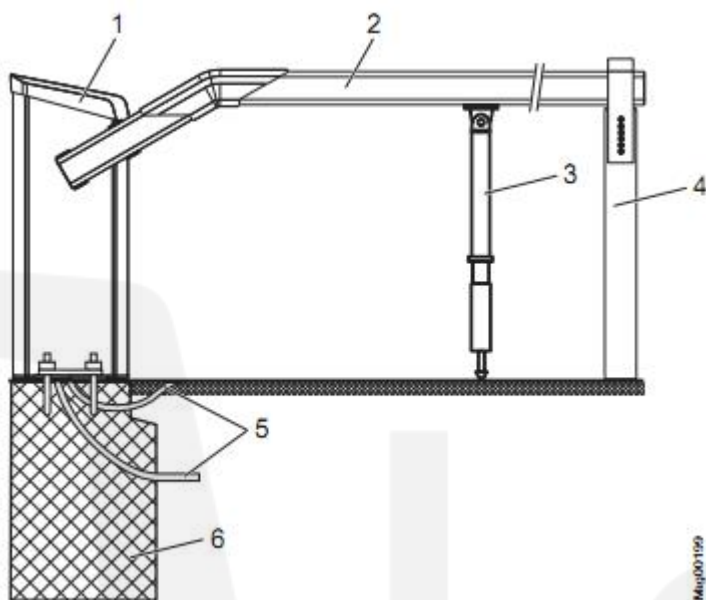
图 7：栏杆系统“Access”系列和“Parking”系列
