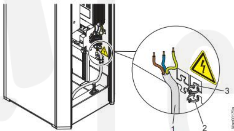
图 38 安置电源线
