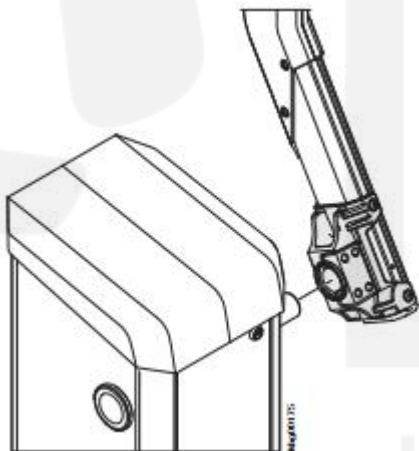
图 53：从栏杆臂上拆下回转
