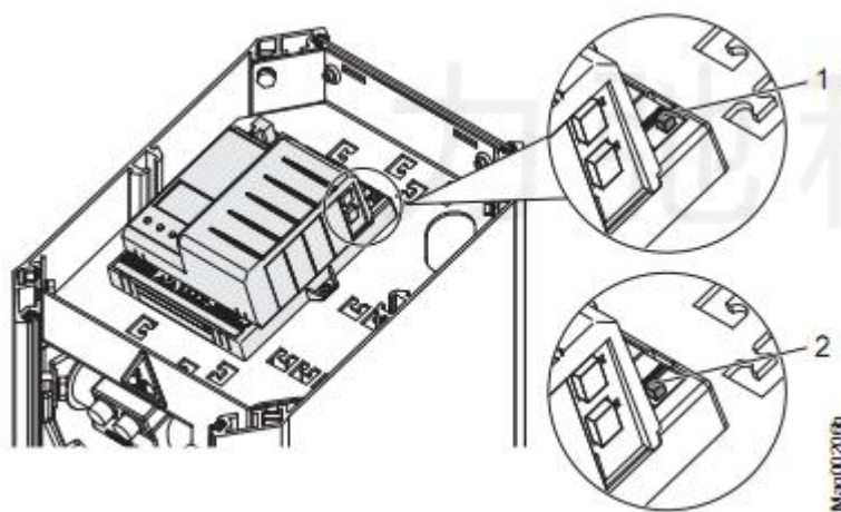
图 46: 测试开关
