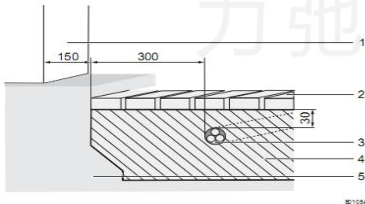
图 23 在锁石铺设的路面安装感应线圈
