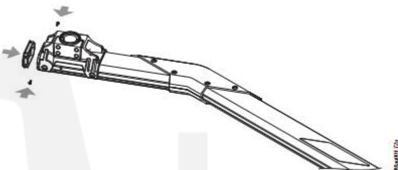
图 30 安装端盖 9. 将事先安装好回转的栏杆臂安装在主轴上。
