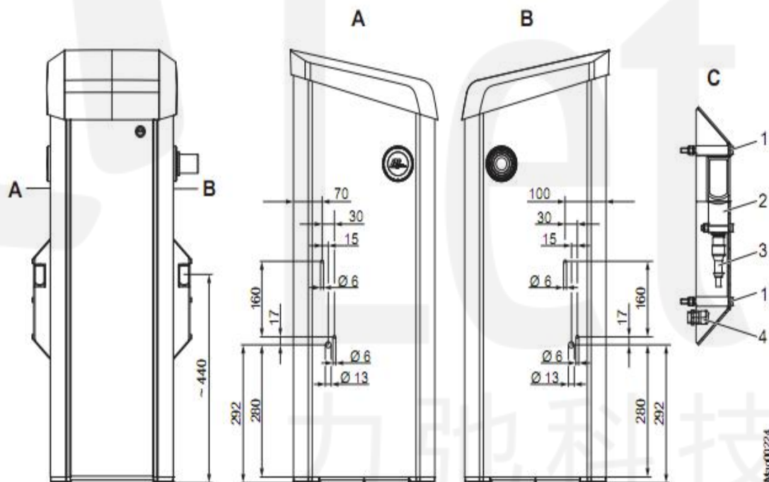
图 25 栏杆机箱上发射器的光栅机箱的安装。
