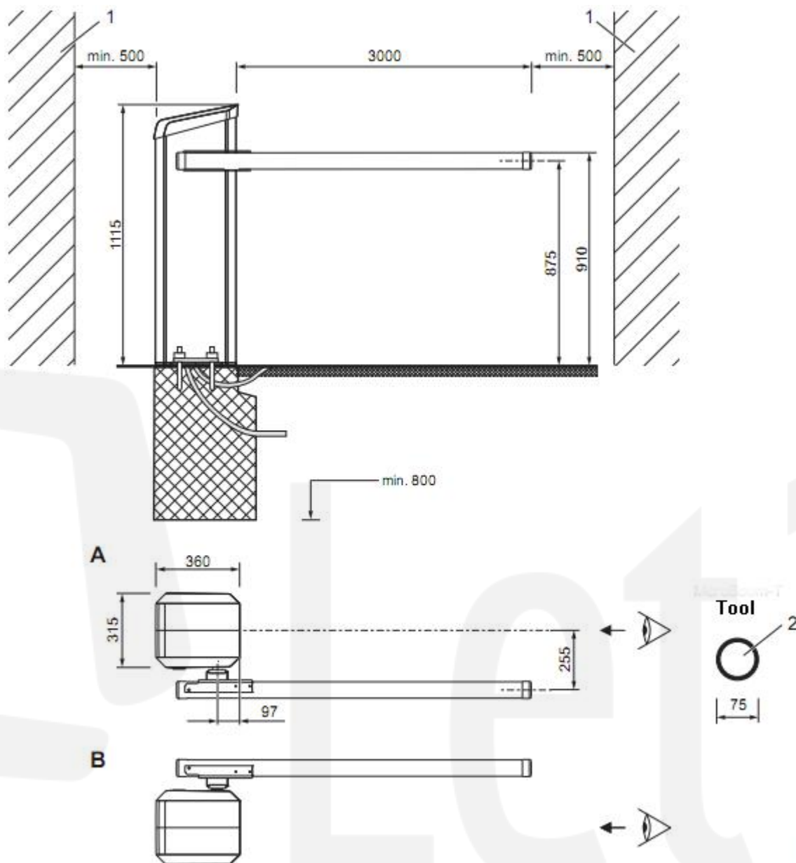
图 6: 栏杆机系统尺寸和栏杆臂简介——“Toll”系列
