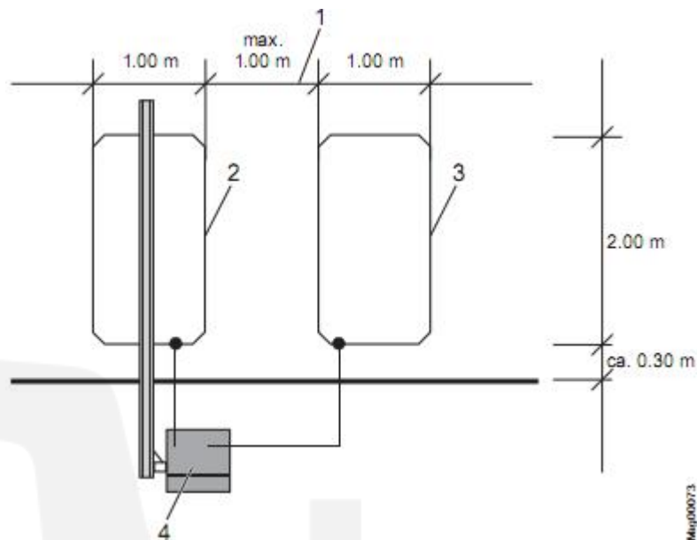
图 10: 客车感应线圈
