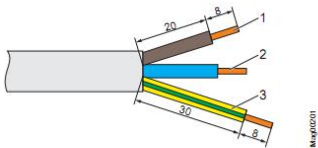
图 37: 剥电源线。
