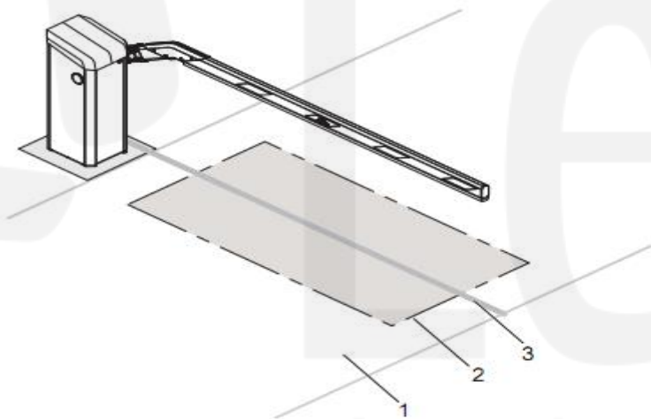
图 20 用于客车的线圈部署
