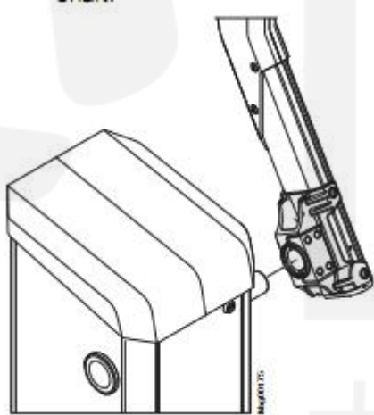
图 31: 安装带有栏杆臂的回转
