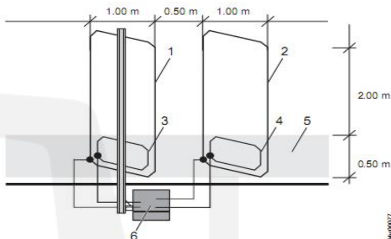
图 14：客车和摩托车线圈
